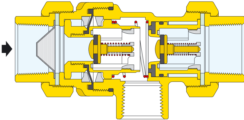
VENT
