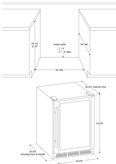
Figura A – La profundidad del recorte debe ser el 24"
