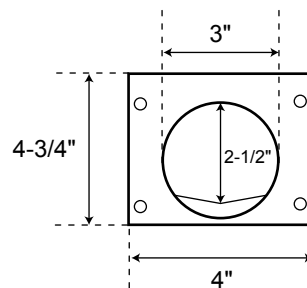
Outlet End
